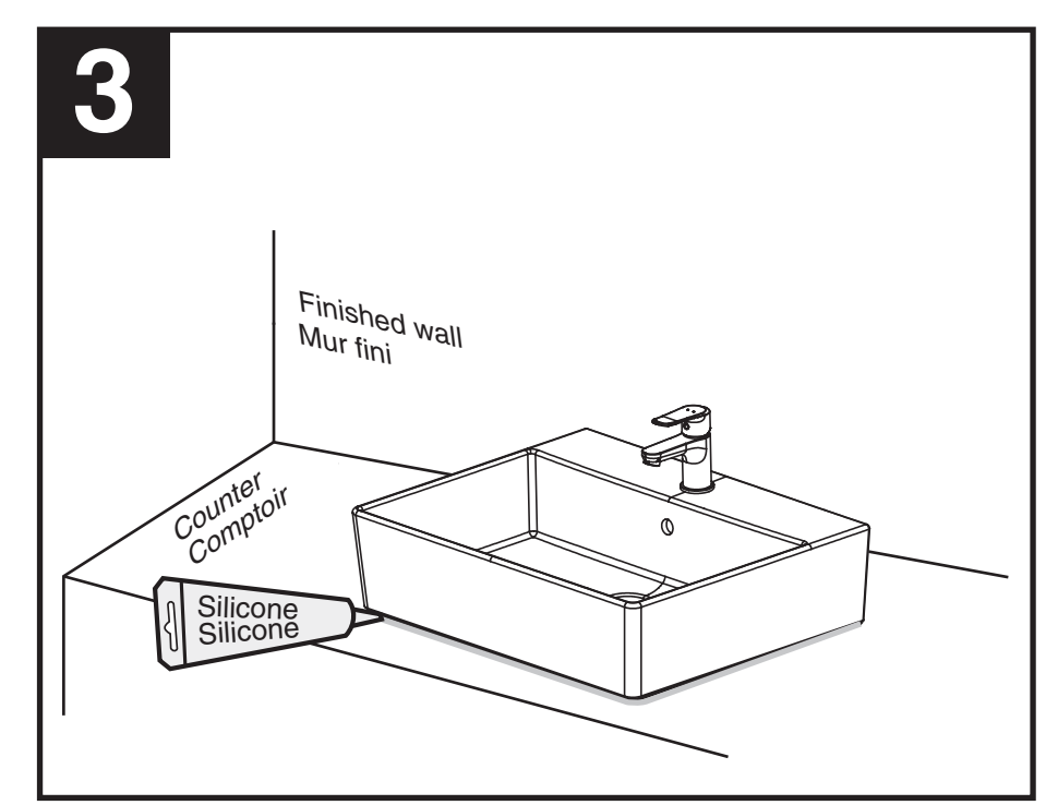
Set the vessel on the counter. Connect the drain. Apply silicone to seal the gap around the vessel. (Sealing material is not provided.) Placez le lavabo sur le comptoir. Raccordez le renvoi. Appliquez du silicone afin de sceller l'écart autour du lavabo. (Le scellant n'est pas fourni.)
